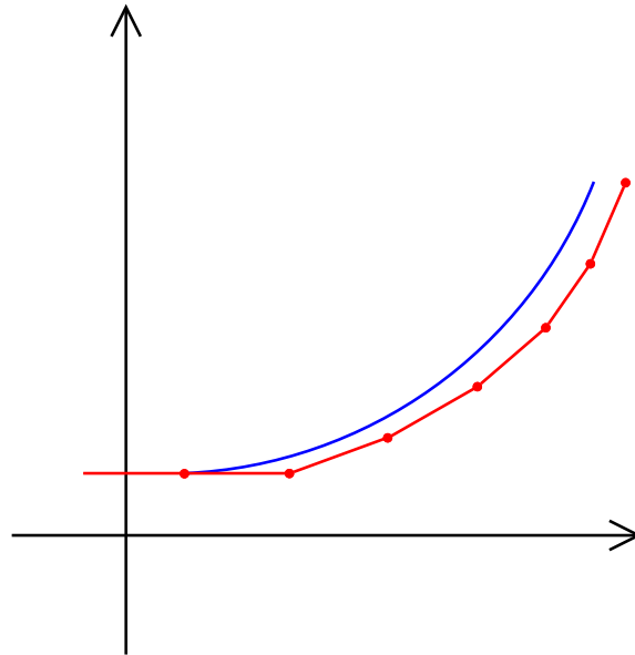
Figur 5.1: Illustrasjon av Eulers metode. For hvert nye steg går metoden en viss lengde langs tangenten. Den røde linjen illustrerer funksjonen approksimert med Eulers metode mens den blå linjen er den eksakte funksjonen.
