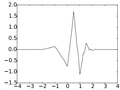
(d) \psi for N=3
