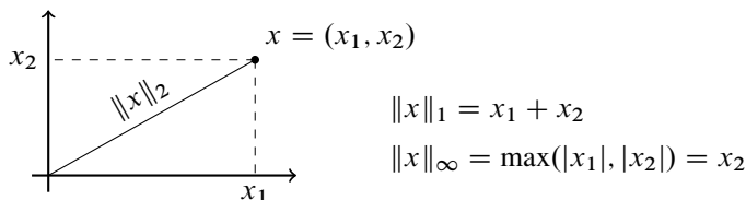
Figur 3.1: p -normene i \mathbb{R}^2 . Merk at siden x ligger i første kvadrant, er både x_1 og x_2 ikke-negative, slik at vi kan fjerne absoluttverditegnene.
