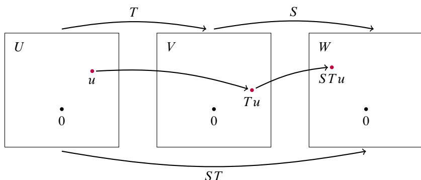
Figur 2.1: Lineære avbildninger T \in \mathcal{L}(U, V) og S \in \mathcal{L}(V, W) .
