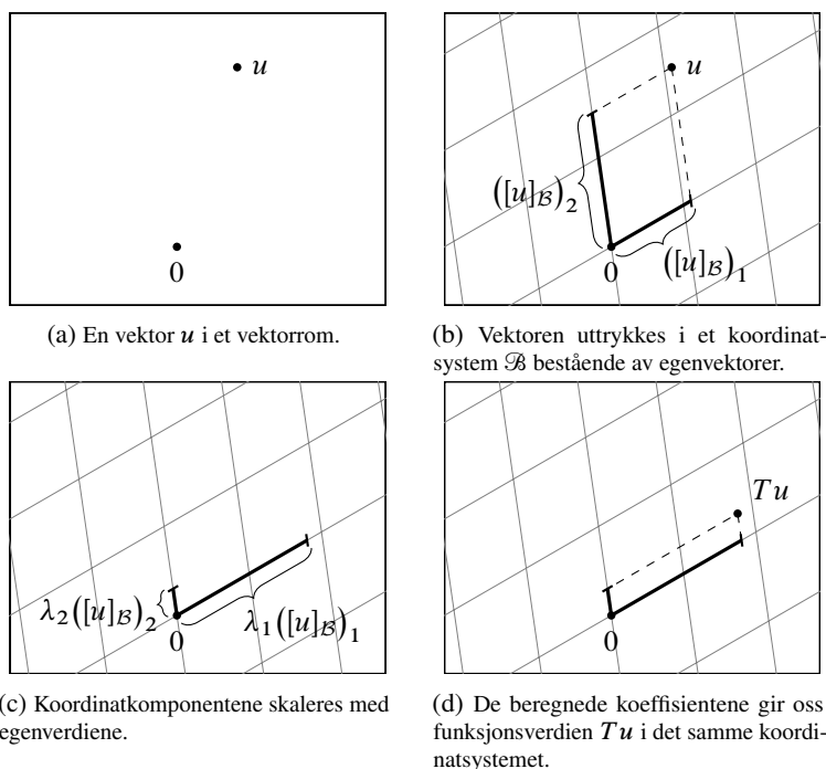
Figur 5.1: Illustrasjon av en diagonaliserbar operator T .
